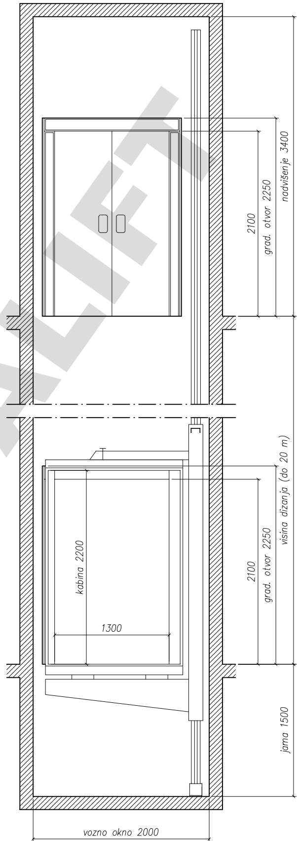
PRESJEK B-B
